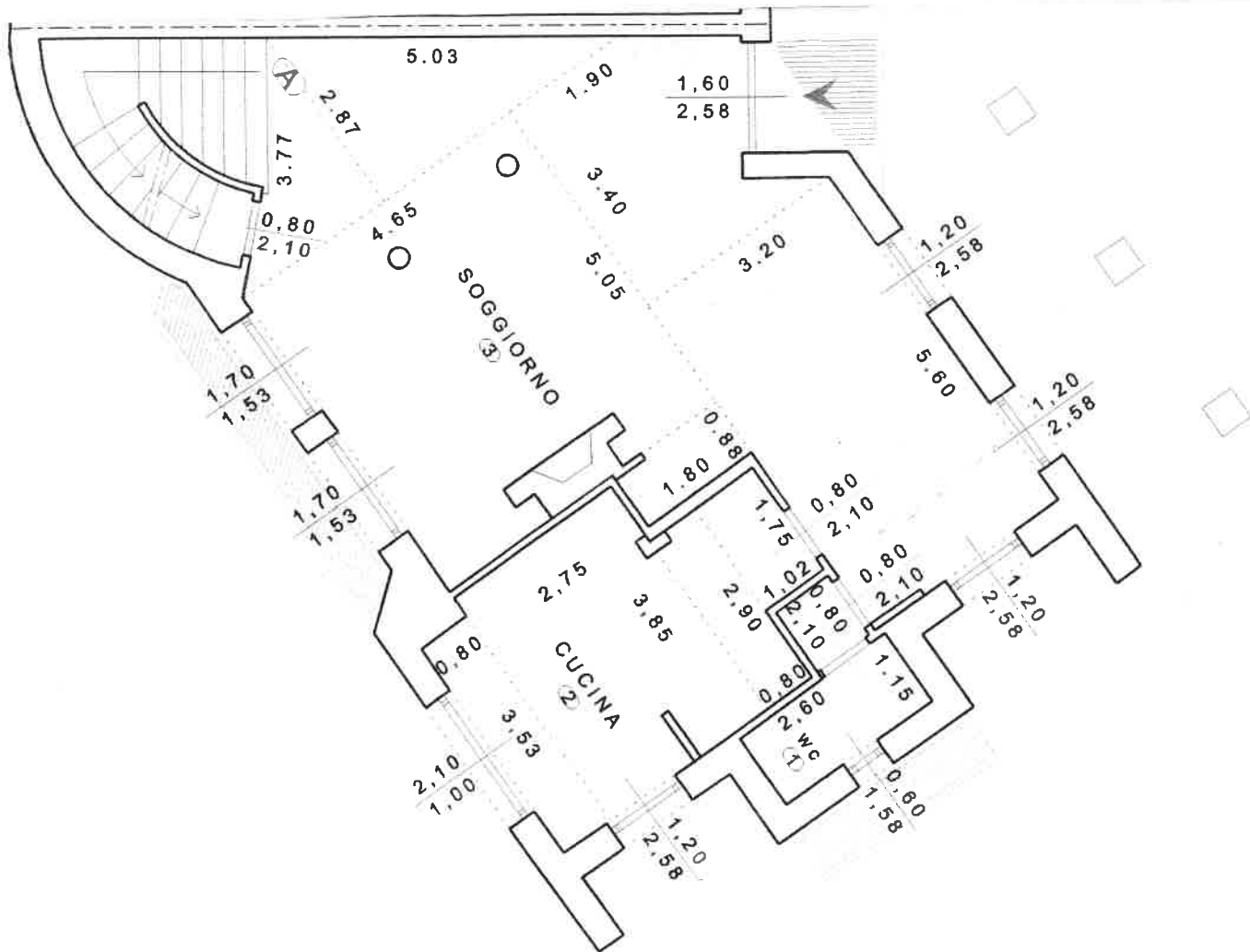
- PIANTA PIANO TERRA I
